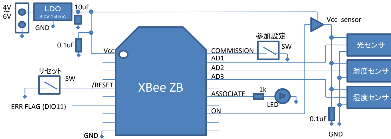
「ZB Coordinator」対応センサーの回路図
